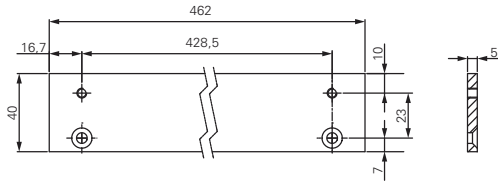
Adaptionsprofil für Gleitschiene HG
