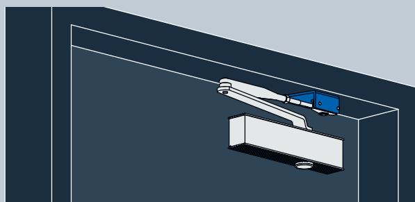
Befestigungswinkel Parallelarmmontage Gelenkarmschließer
