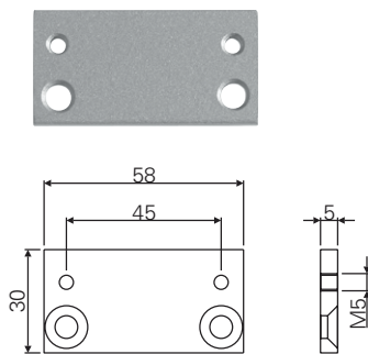
Adaptionenprofil für Gelenkarmschließer
