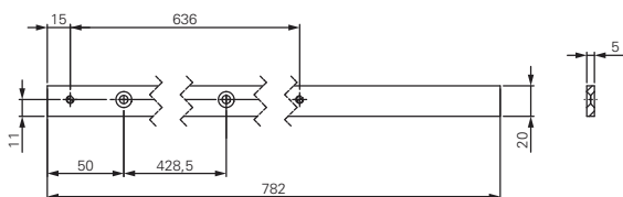
Adaptionsprofil ADP 20 für Gleitschiene SR III
