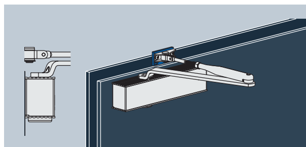
Adaptionenprofil zur Normalmontage Gelenkarmschließer
