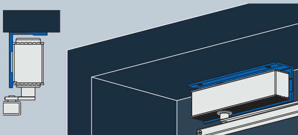
Sturzfutterwinkel zur Kopfmontage Gelenkarmschließer (links) bzw. Gleitschienenschließer (rechts)
