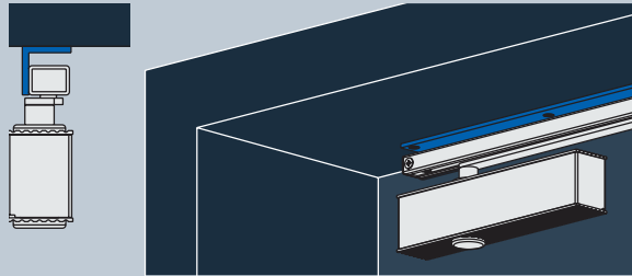
Sturzfutterwinkel zur Normalmontage Gleitschienenschließer
