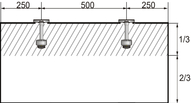
Anordnung des Rauchschalters mit dem Sockel 164 K im Lüftungskanal
