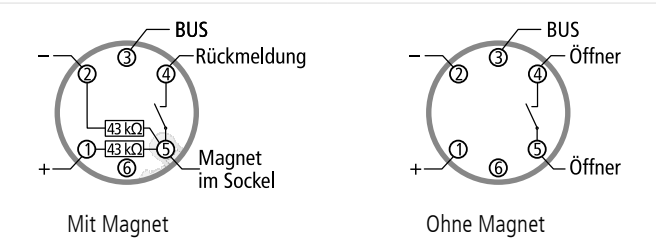
Interne Beschaltung
