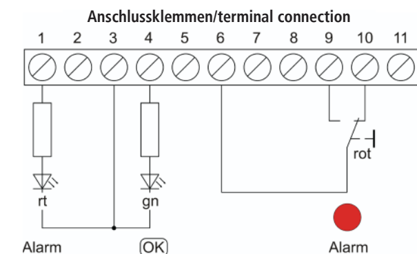
Anschluss/Verdrahtung Connection/wiring
