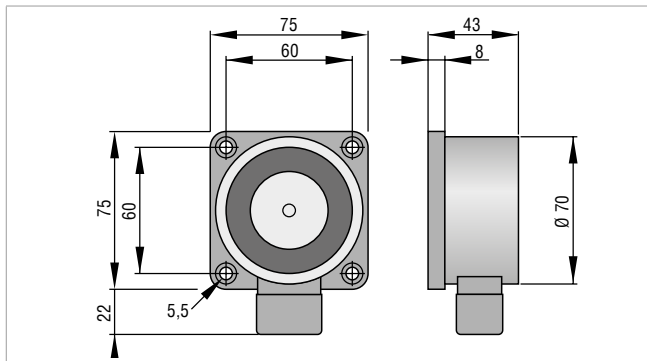
Haftmagnet THM 425-1
