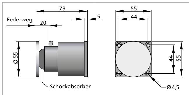
Teleskopanker ATS 55
