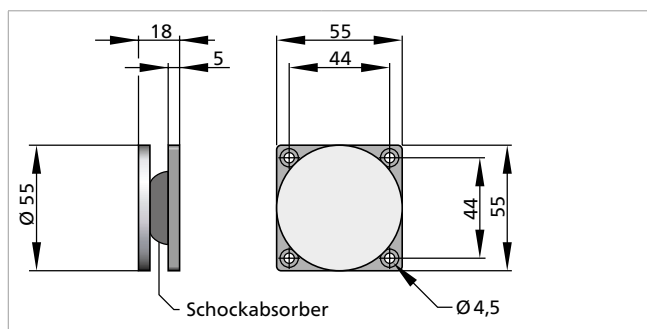
Standardanker ASS 55
