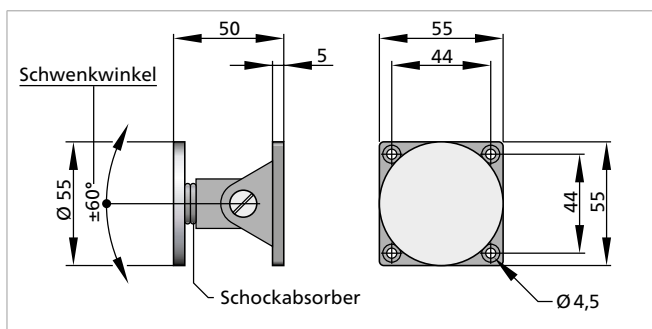
Flexibler Anker AFS 55
