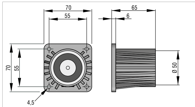
Haftmagnet THM 440
