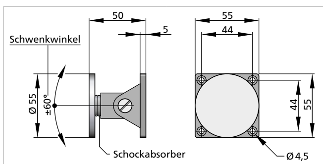
Flexibler Anker AFV 55
