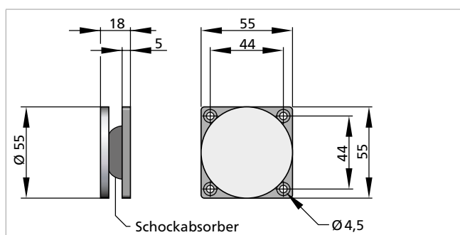
Standardanker ASV 55
