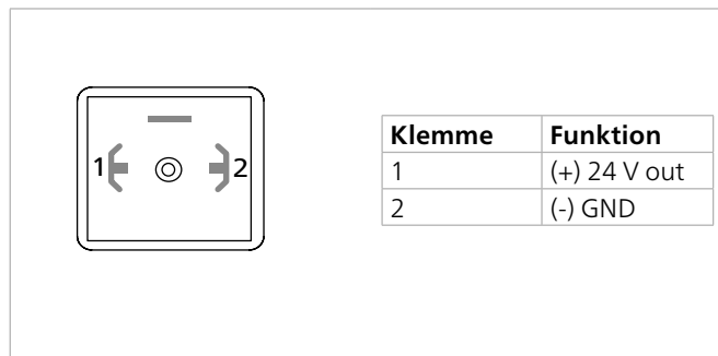
Anschlussklemme
