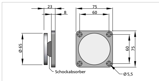
Standardanker ASV 65
