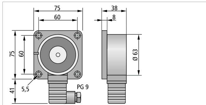
Haftmagnet THM 442
