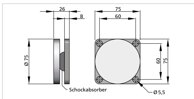
Standardanker ASV 75
