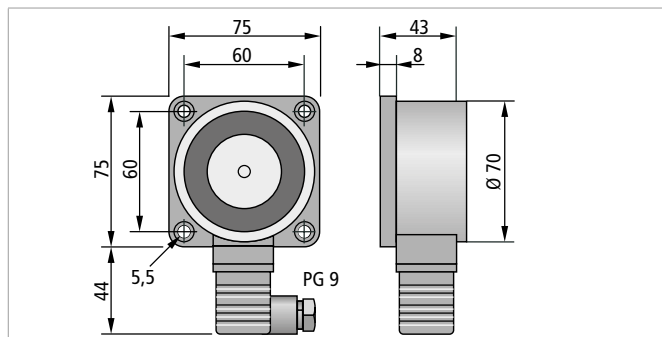
Haftmagnet THM 443
