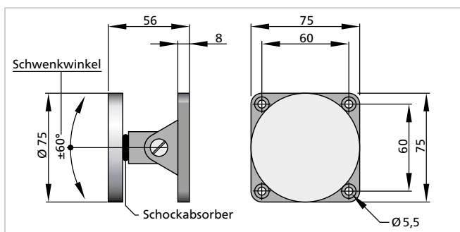
Winkelanker AFV 75
