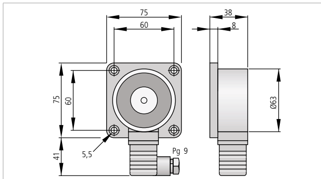
Haftmagnet THM 446
