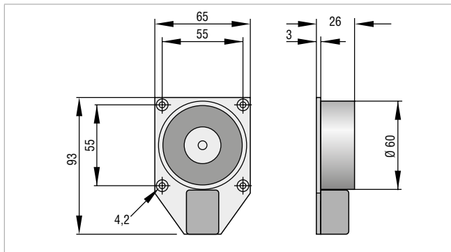
Haftmagnet THM 425
