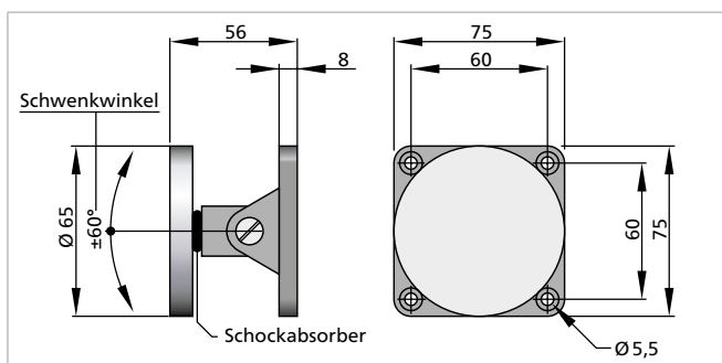
Winkelanker AFS 65
