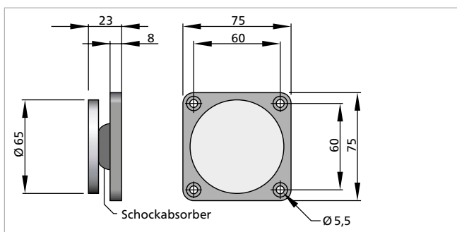
Standardanker ASS 65
