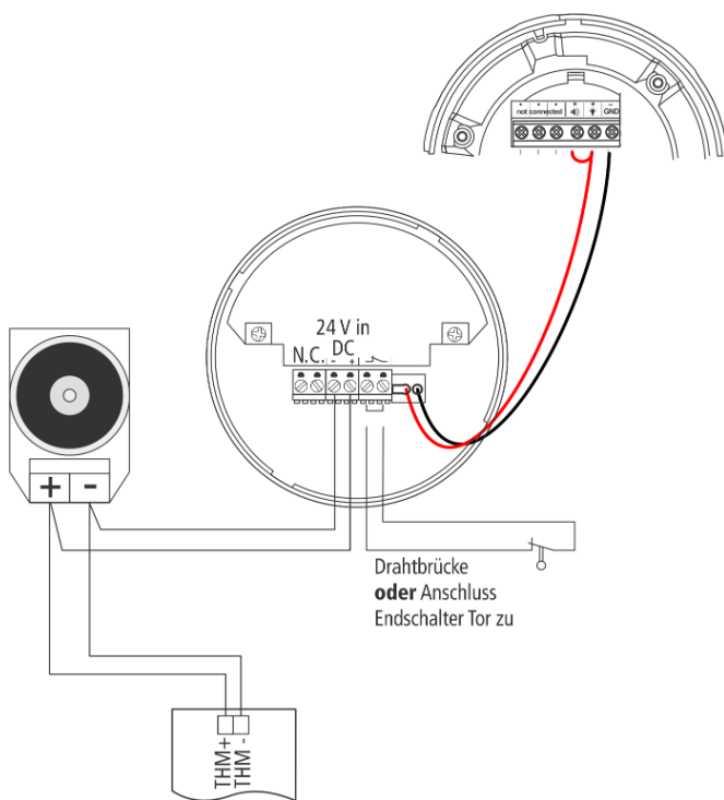
Abb. 3: Anschlussbeispiel
