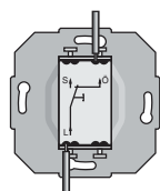
Anschlussschema als Öffner
