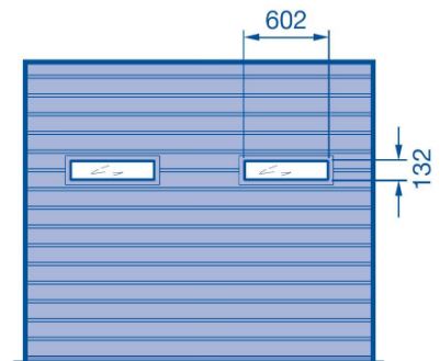
Verglasung Typ D
