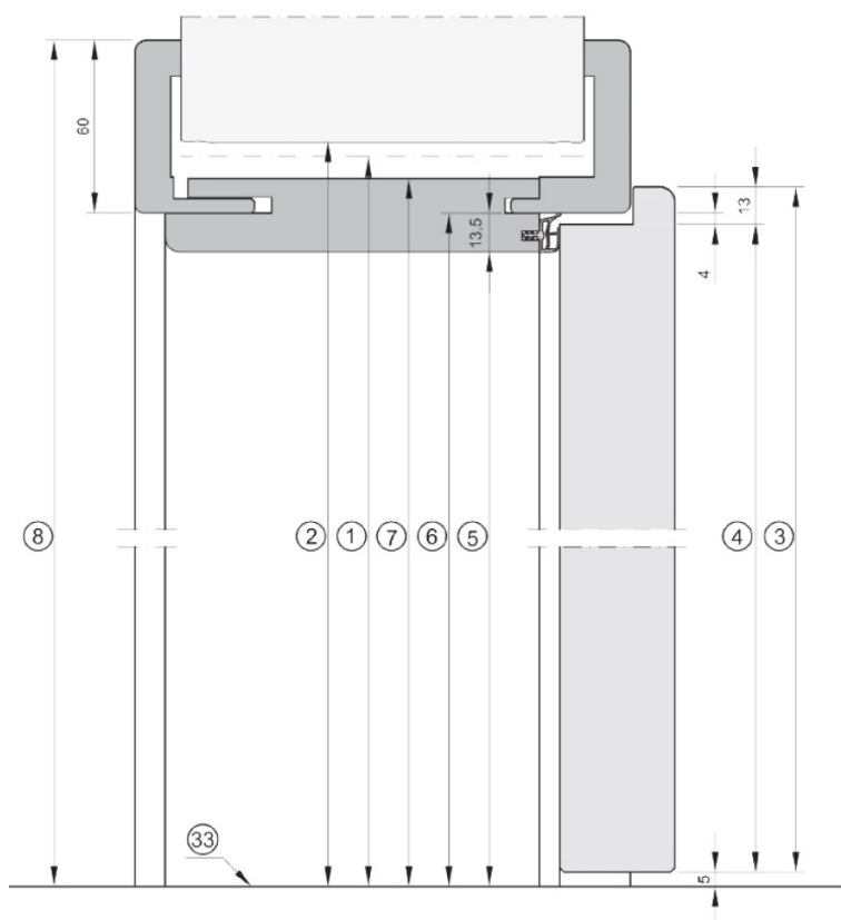
Maßtabelle Breite
