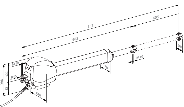
Abmessungen Motor-Aggregat, Ausführung lang
