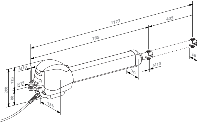
Abmessungen Motor-Aggregat, Ausführung lang
