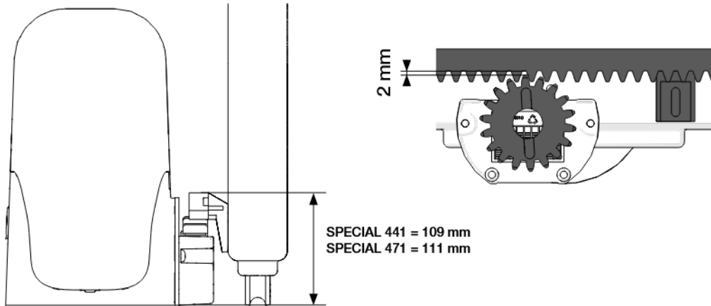
Fig. 10 IT - Fissaggio cremagliera EN - Rack assembling FR - Pose de la crémaillère ES - Fijación de la cremallera
