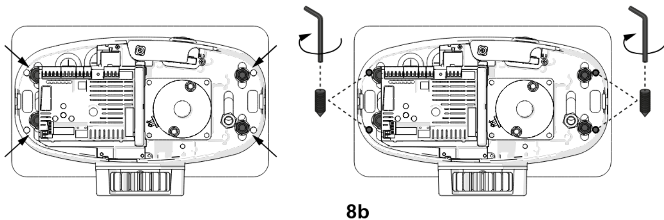
Fig. 9 IT - Chiusura del coperchio EN - Closing the cover FR - Fermeture du couvercle ES - Cierre de la tapa
