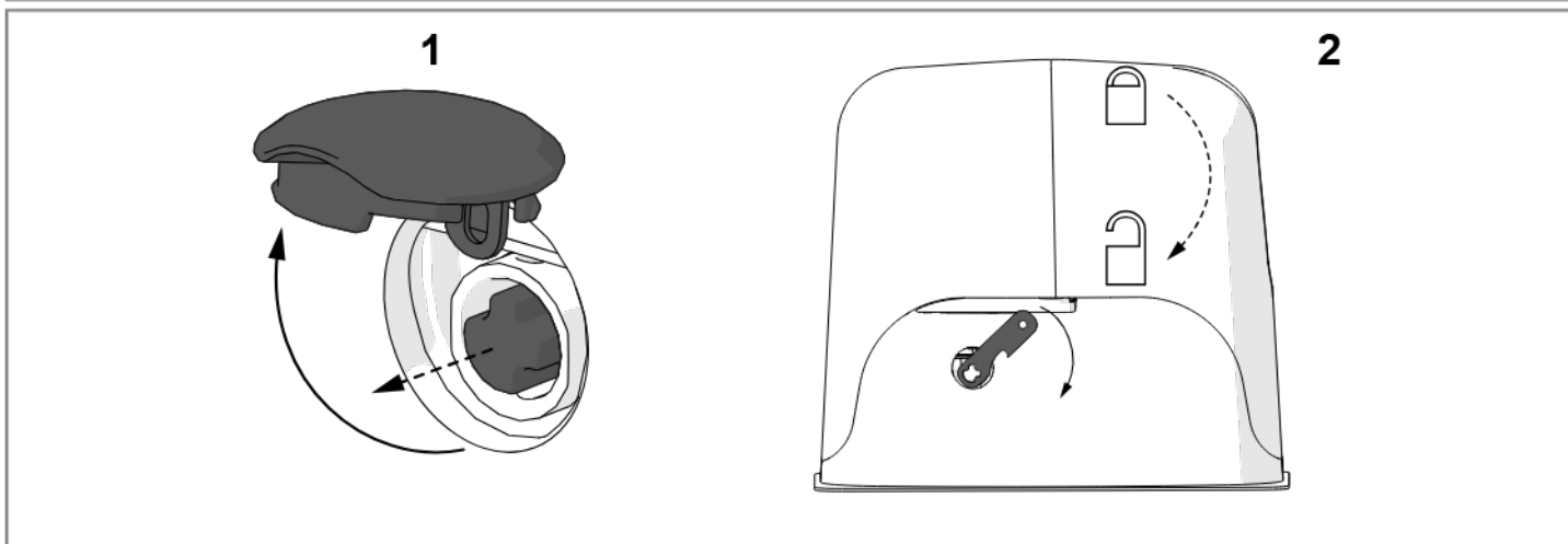
Fig. 4 IT - Sblocco del motoriduttore EN - Gearmotor release FR - Débloçage du motoréducteur ES - Desbloqueo del motorreductor
