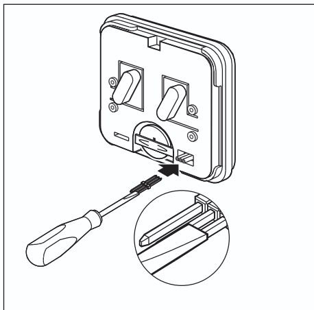
Fig. 8: Modifier le codage 1 + 2
