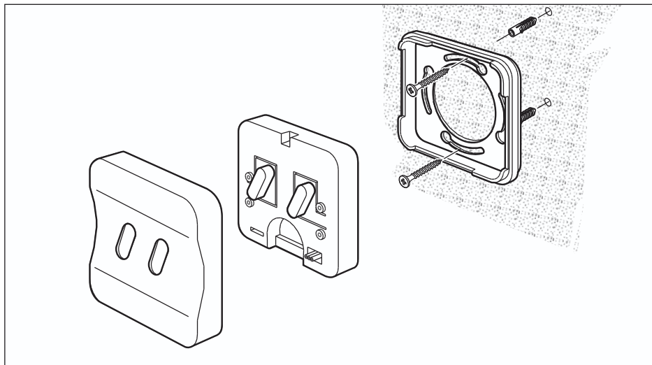
Fig. 3: Montage
