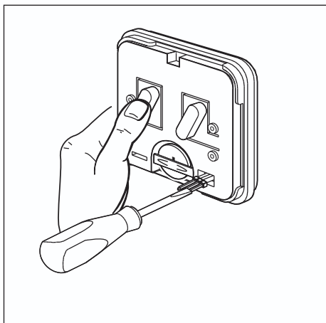
Fig. 9: Modifier le codage - 3
