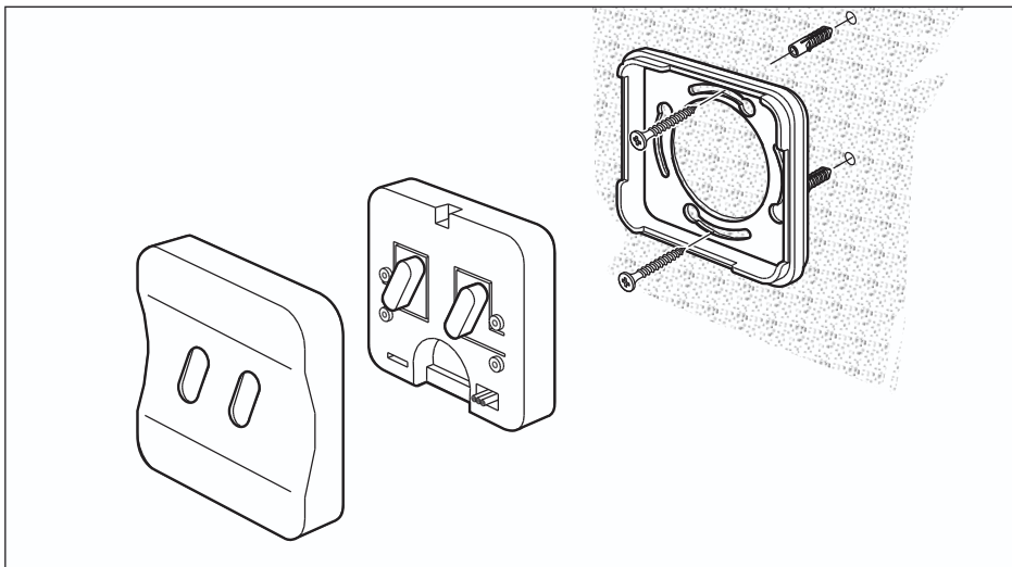
Afb. 3: Montage
