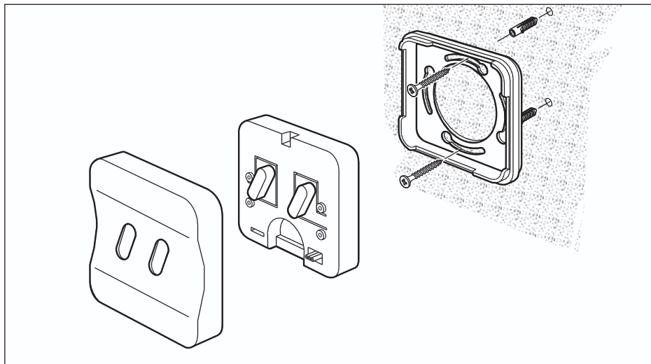
Abb. 3: Montage
