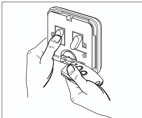
Fig. 6: Apprendre le codage -3
