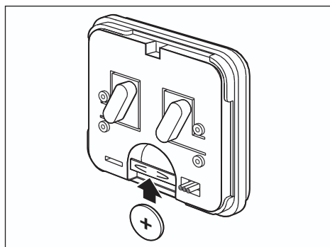
Afb. 2: Batterijen plaatsen
