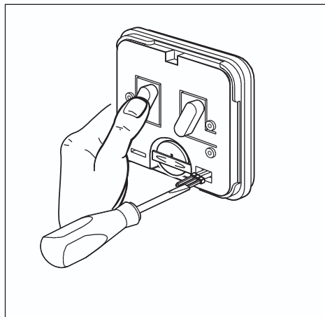
Abb. 9: Codierung ändern - 3
