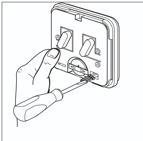
Fig. 10: Modifier le codage -4
