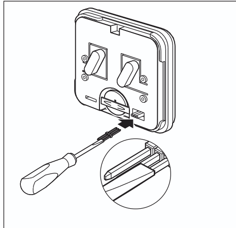
Afb. 8: Code veranderen - 1+2
