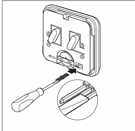
Abb. 8: Codierung ändern - 1+2
