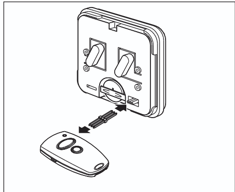
Abb. 4: Codierung lernen - 1
