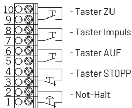
Befehlsgeräte
