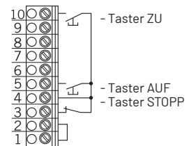
Taster AUF / STOPP / ZU (4-Ader Lösung)
