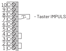
Taster IMPULS
