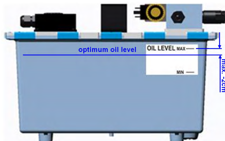
Optimaler Ölstand in Ruhelage (max. -2cm unter „OIL LEVEL MAX“)
