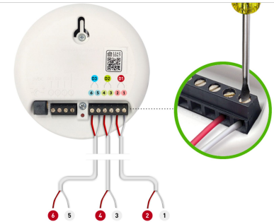
Installation für 3 Tore
