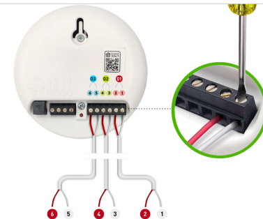
Installation für 3 Tor
