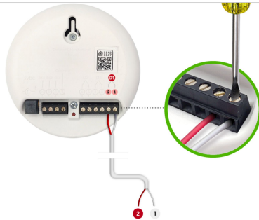
Installation für 1 Tor
