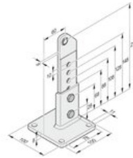
Torpfostenbeschlag mit Kugelgelenk 60/210 L
