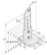
Torpfostenbeschlag mit Kugelgelenk 60/210 R
