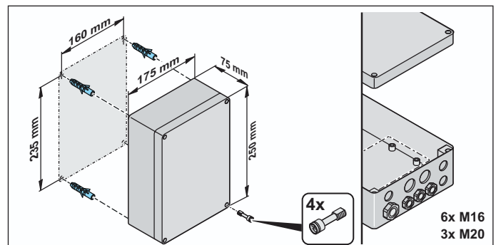
Abb. Montagebeispiel zur Befestigung der Steuerung
