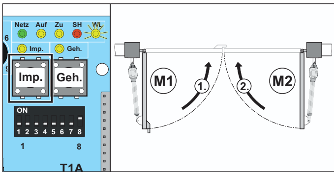
Abb. Tor ZU
