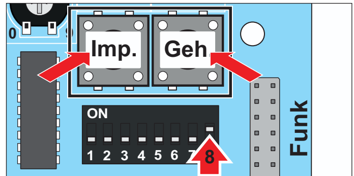
Abb. Taster (Imp. + Geh.)
